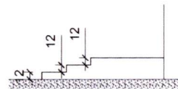
Przekrój A-A
